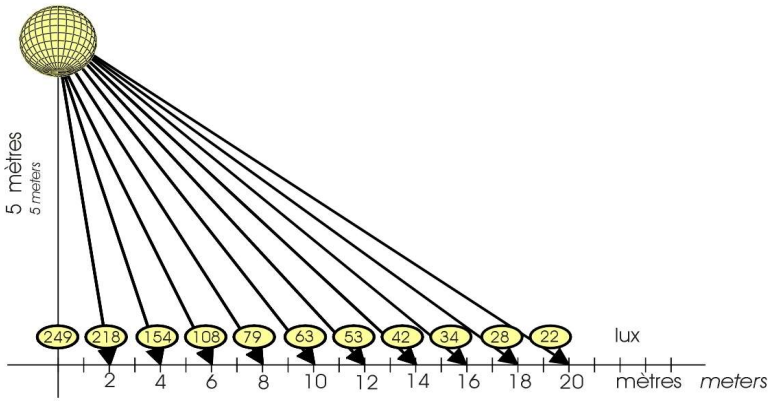
Flux lumineux Lunix 200 Halogène
