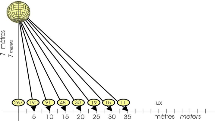
Flux lumineux Lunix 370 Halogène
